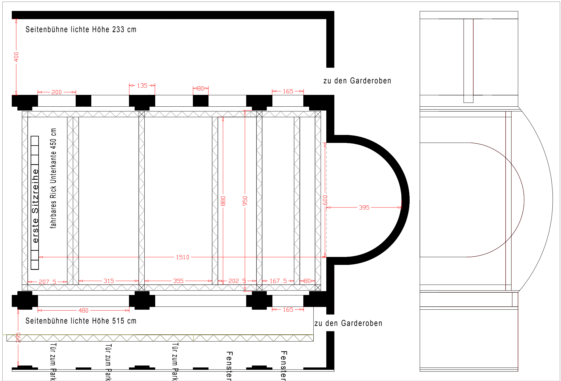
Technische Zeichnung Bühne Maß in cm
